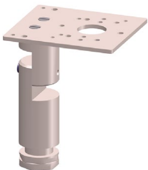
Adapter Pyranometer verstellbar
